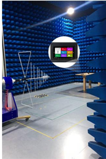
图 5-5 辐射测试图
