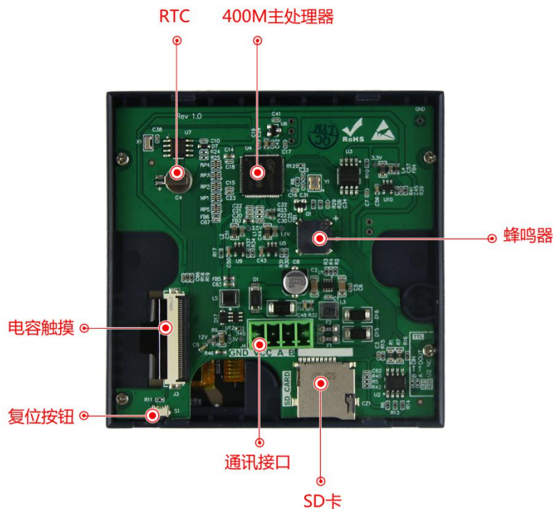
图 1-2 硬件配置图
