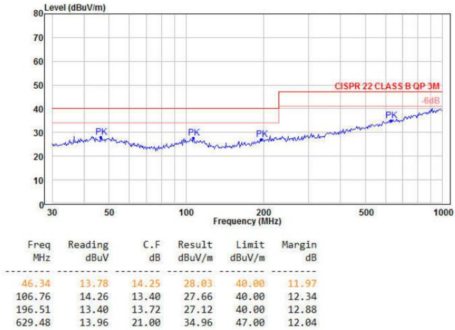
图 5-7 辐射测试垂直方向
