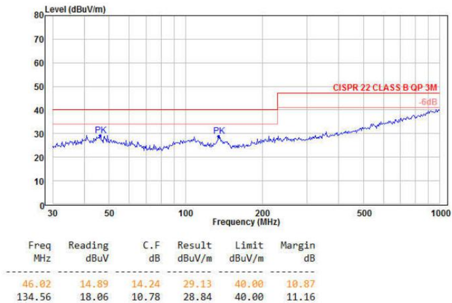
图 5-6 辐射测试水平方向
