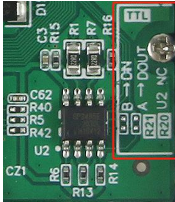
图 7-1 RS485 和 TTL 转换电路
